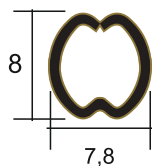
Профиль FBS 1062 не перфорированный Материал: алюминий Размер: 8 мм x 8 мм Цвет: белый, золото, хром
