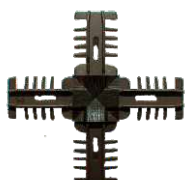
Крестовое соединение Материал: пластик Размер: 8 мм x 18 мм/8 мм x 25 мм Цвет: темный дуб
