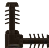
L-образная деталь для соединения раскладки Материал: пластик Размер: 8 мм x 18 мм/8 мм x 25 мм Цвет: белый, коричневый
