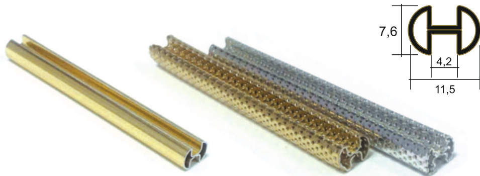
Профиль FBS 1156 не перфорированный под стекло 4 мм Материал: алюминий Размер: 7,6 мм x 11,5 мм x 4,2 мм Цвет: золотой
