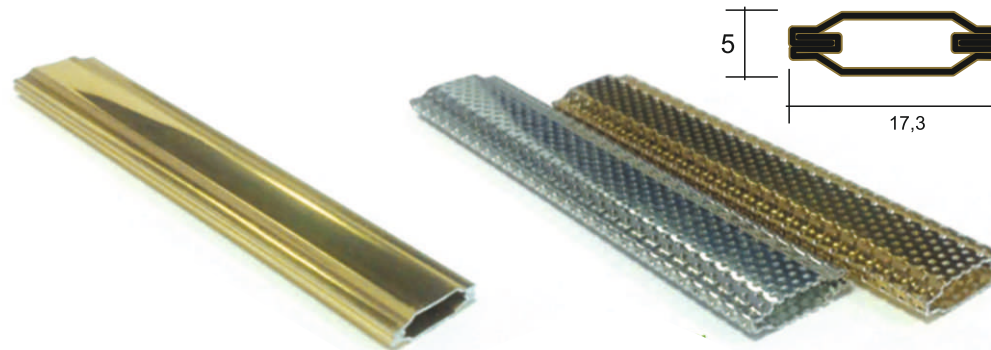
Профиль СЕРИИ FBS 1251 не перфорированный Материал: алюминий Размер: 5 мм x 17,3 мм Цвет: золотой
